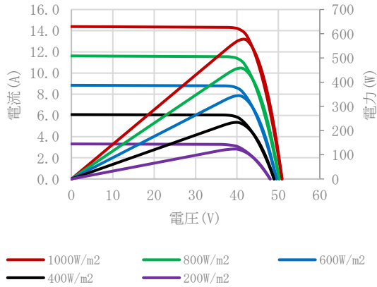
電流-電圧 & 電力-電圧曲線
