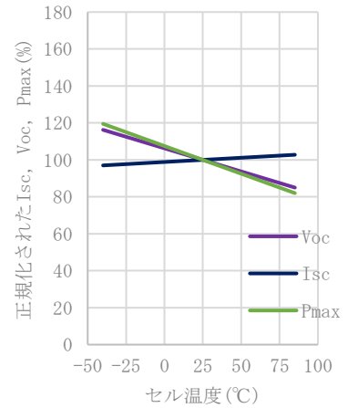
Isc, Voc, Pmax温度依存性
