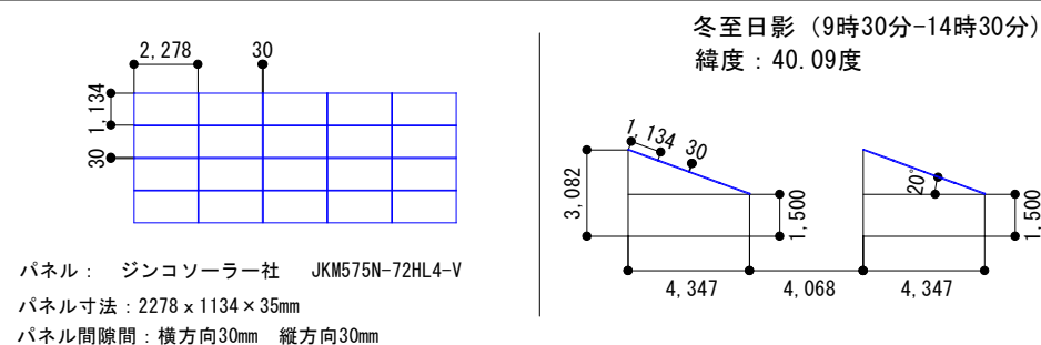
パネルの幅・隙間投影寸法図 パネル勾配20度
