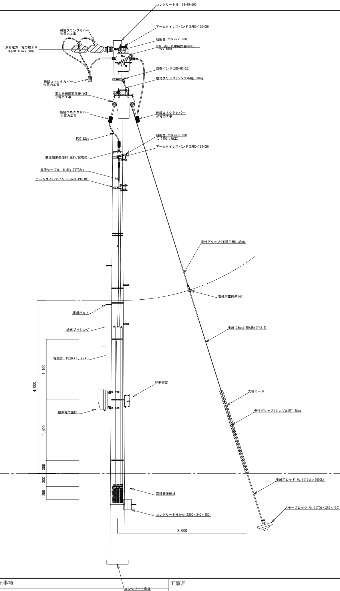
主要設備レイアウト図
